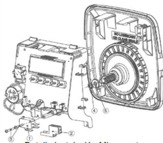
Detalle instalación Micro ruptor
