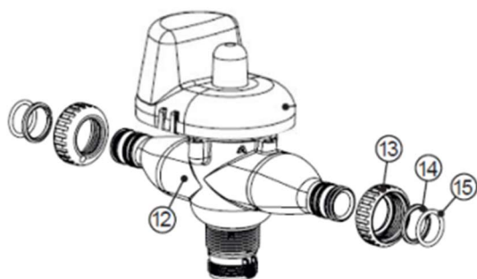
Válvula de 3 Vías "MAV" 1"
