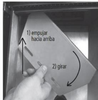
Fig. 17: extracción de la placa cortafuego
