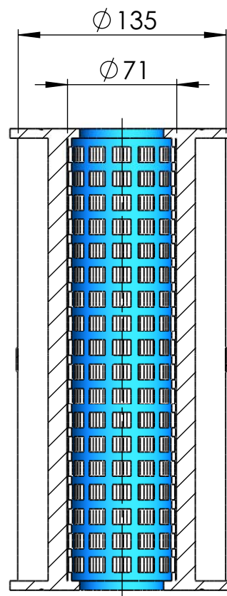
SECCIÓN A-A
