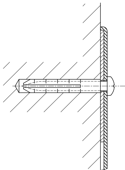
Detalle anclaje Esc. 1:1
