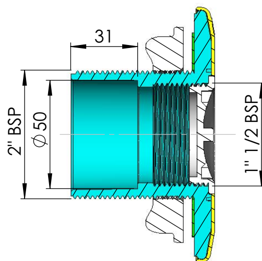
SECCIÓN A-A
