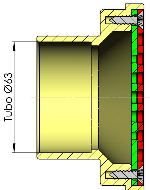
SECCIÓN A-A
