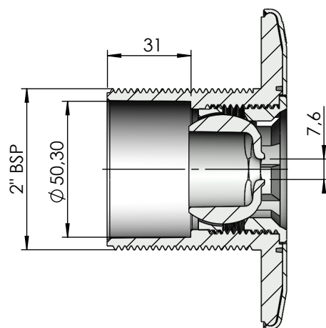
SECCIÓN A-A
