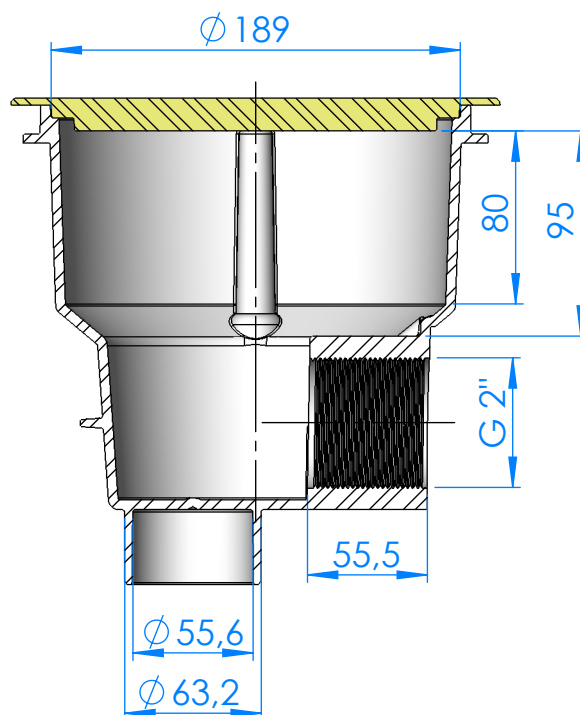
SECCIÓN A-A
